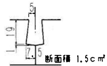
目地詳細図
