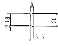
-目地詳細図-
