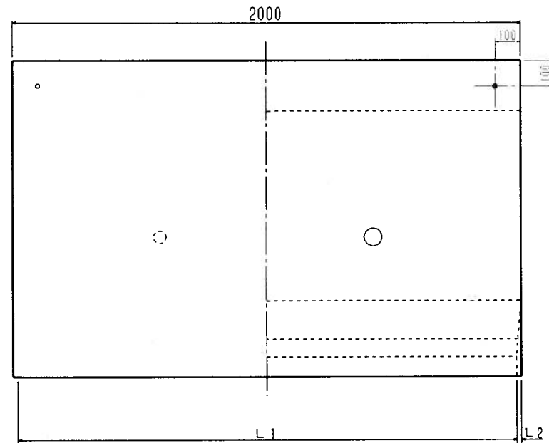
《目地詳細図》
