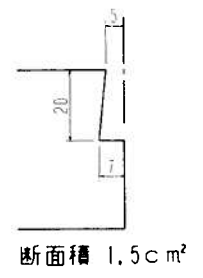
《目地詳細図》
