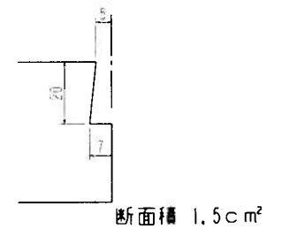
《目地詳細図》
